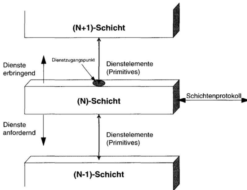
Bild 2 Kommunikation zwischen den Schichten
