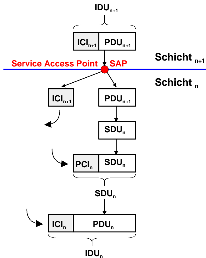
Bild 4 Kommunikation zwischen den Schichten
